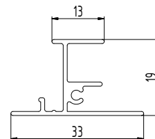
VODICÍ LIŠTA
