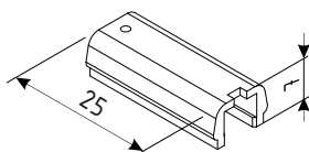
DRŽÁK PROVÁZKU
