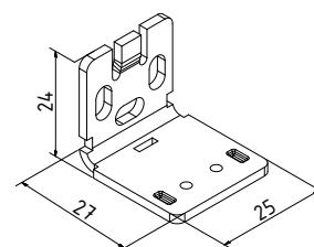
MONTÁŽNÍ KONZOLA
